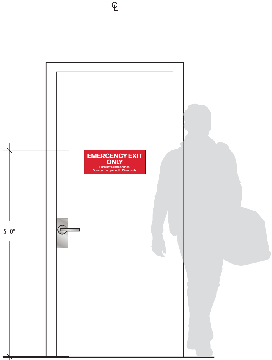
2 ELEVATION SCALE: 3/4" = 1"
