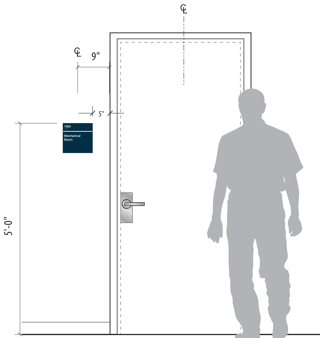
3 ELEVATION SCALE: 3/4" = 1' - 0"
