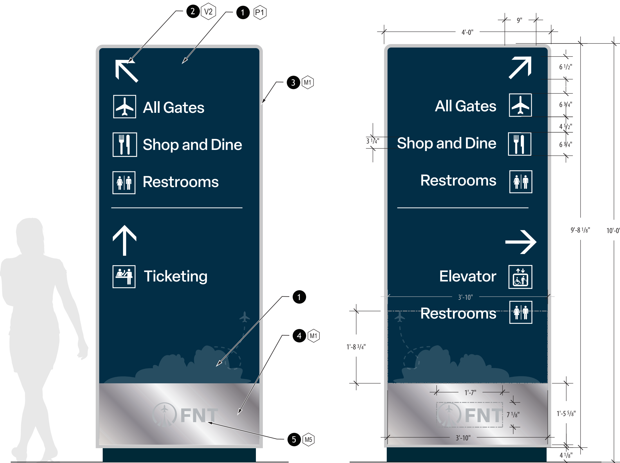
1 SIDE A SCALE: 3/4" = 1"
