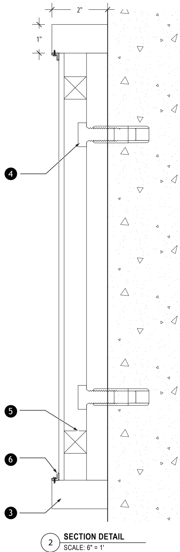
2 SECTION DETAIL SCALE: 6" = 1'
